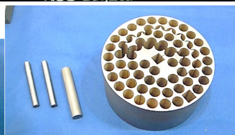
▲SPS 超硬傾斜機能材料とバインダレス超硬 pure-WC 大形焼結体
